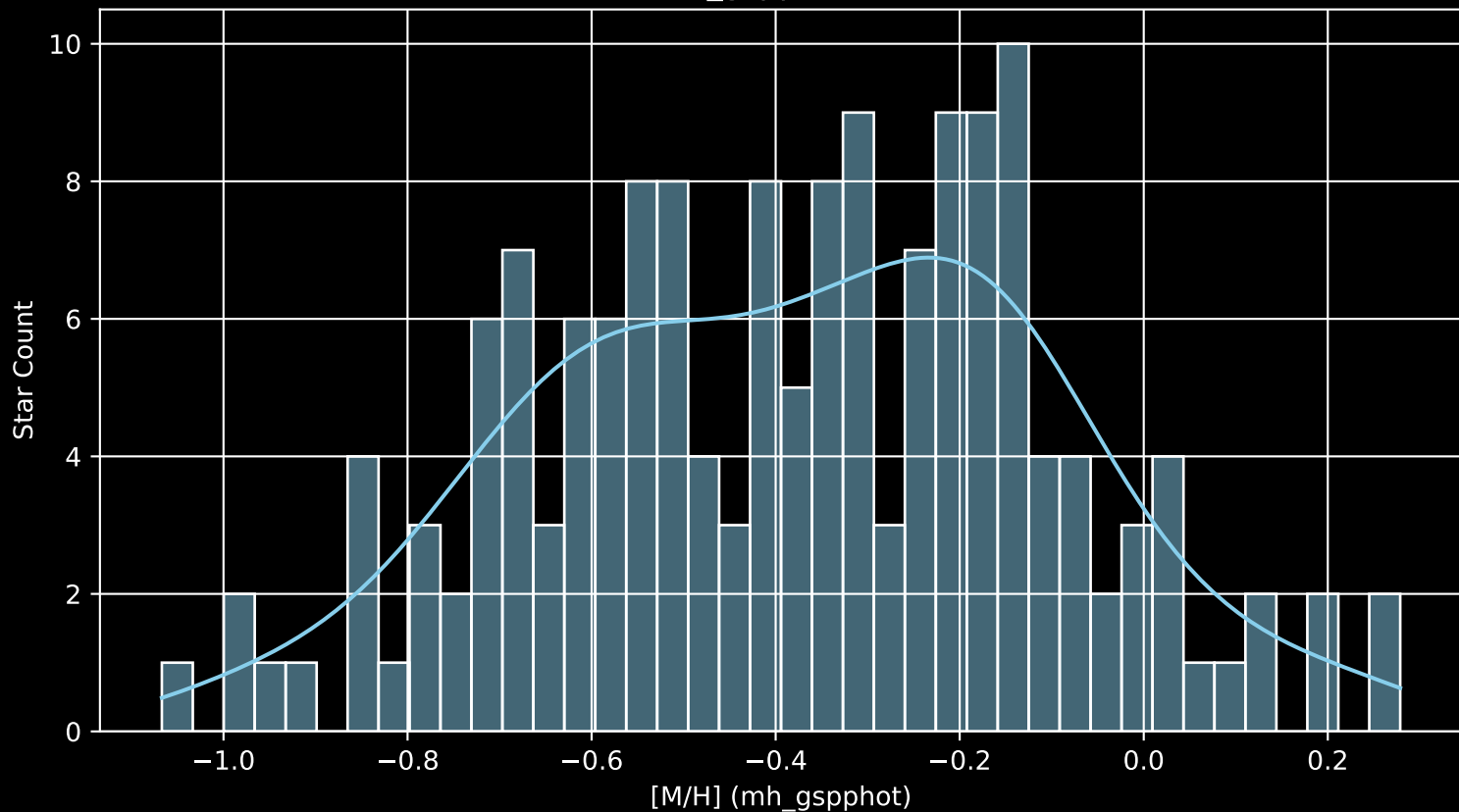
GALAH DR4 Field: [528] [M/H] (mh_gspphot) (n= 159)
