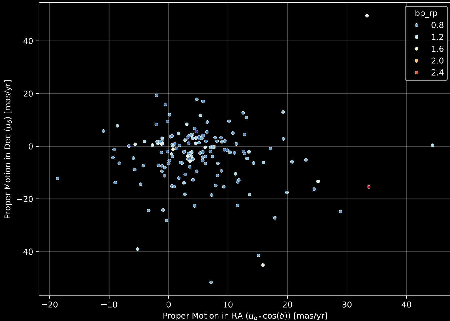
GALAH DR4 Field: [528] Proper Motion Diagram (n= 160)
