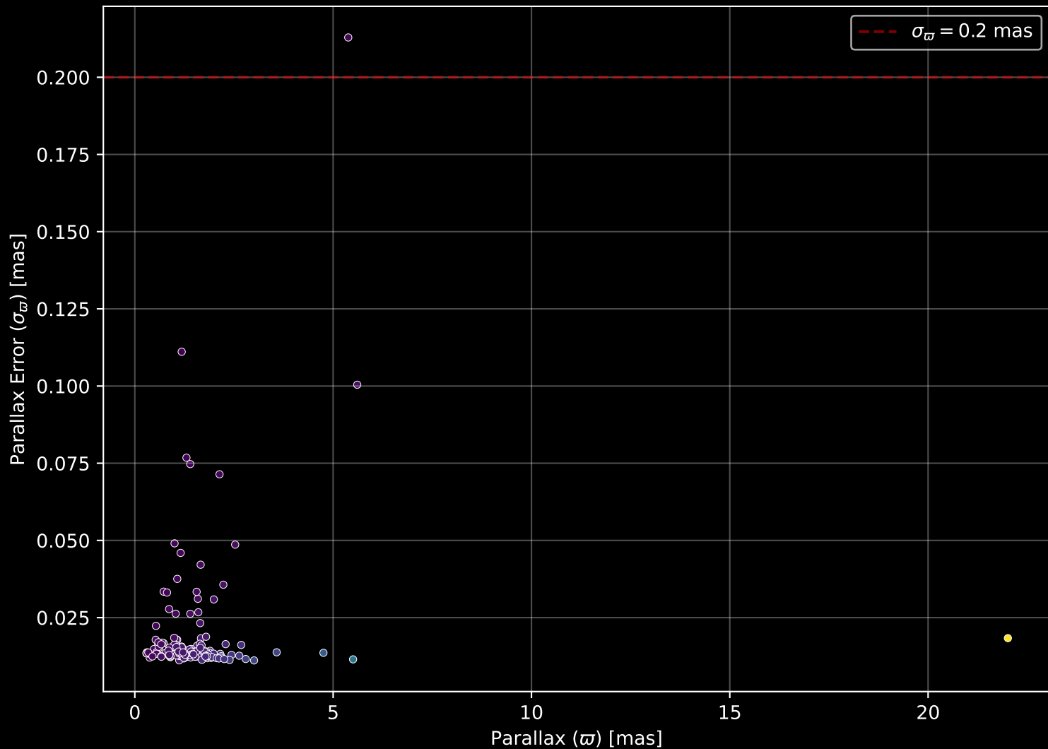
GALAH DR4 Field: [528] Parallax Quality (n= 160)
