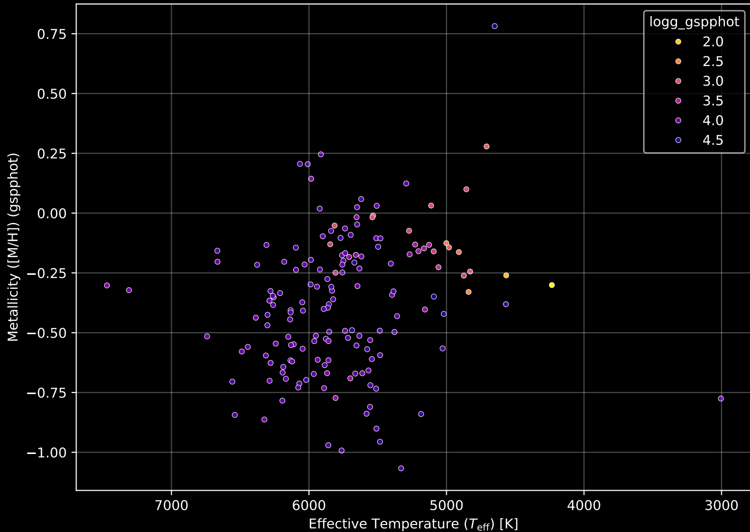
GALAH DR4 Field: [528] Stellar Population Parameters (n= 160)
